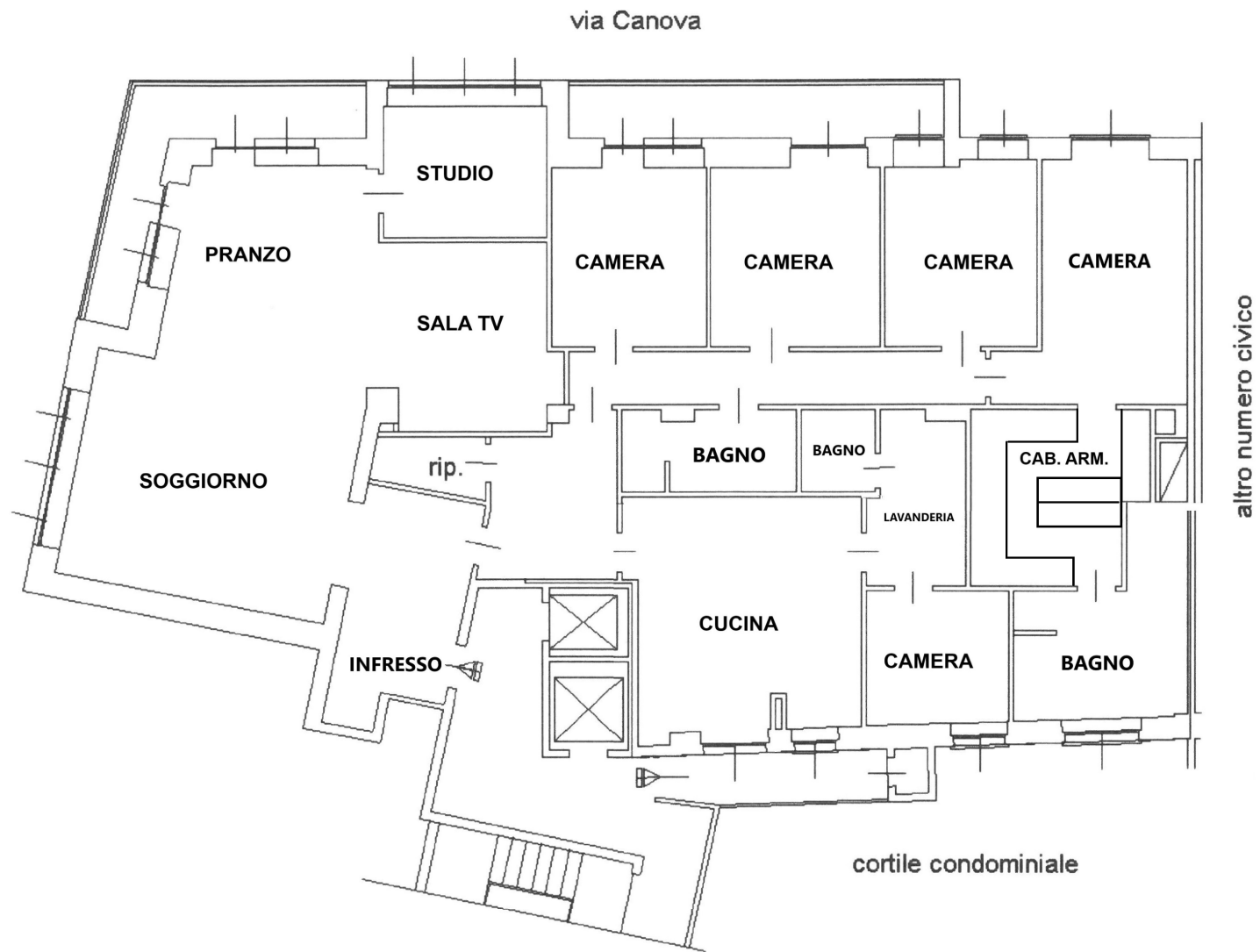
Pianta Piano Secondo H=2.90
